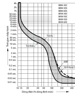
■ Biểu đồ đặc tuyến hoạt động
